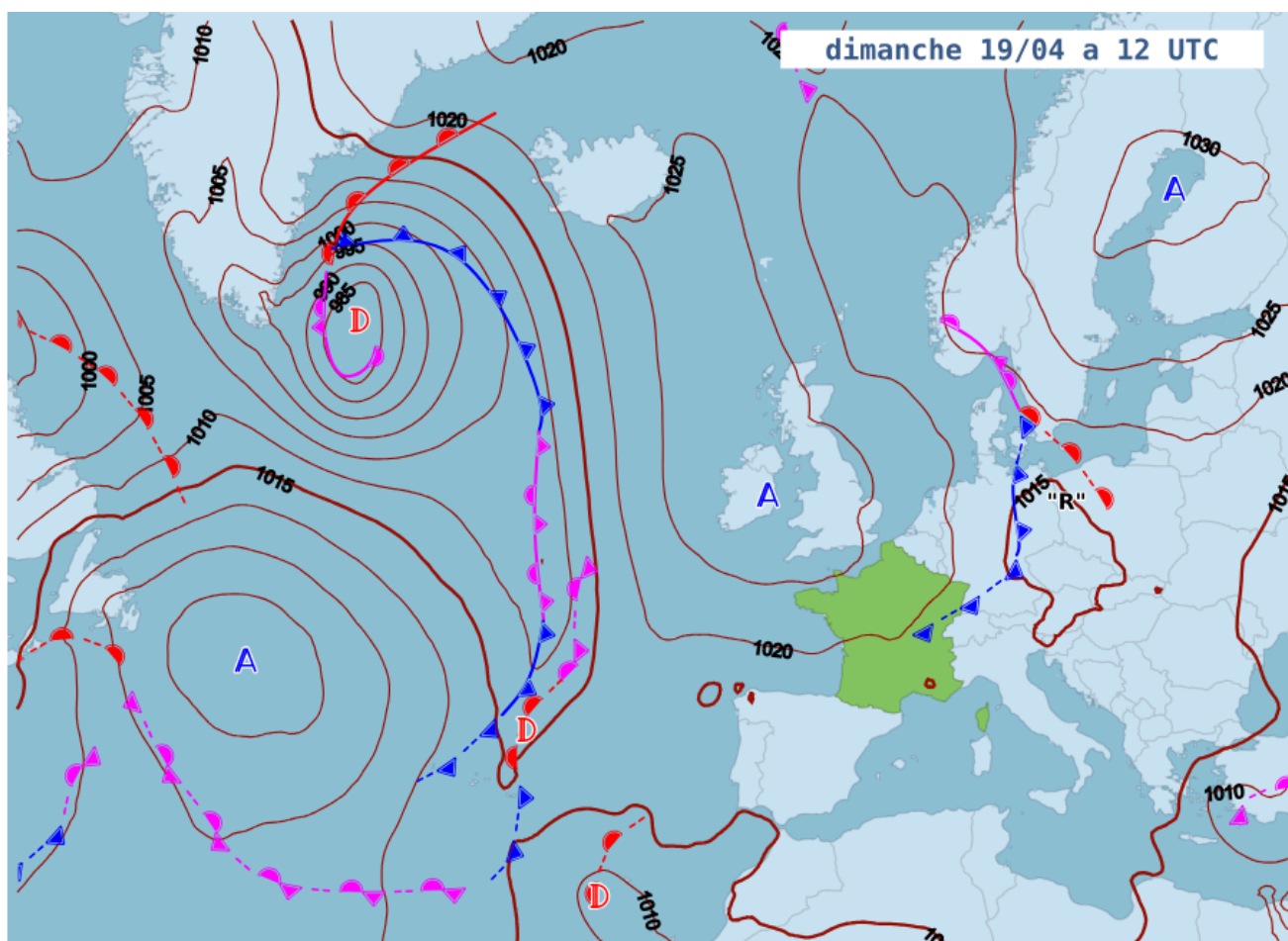
Carte des isobares de pression au niveau de la mer et des fronts prévue pour 19/04 à 14h locales
