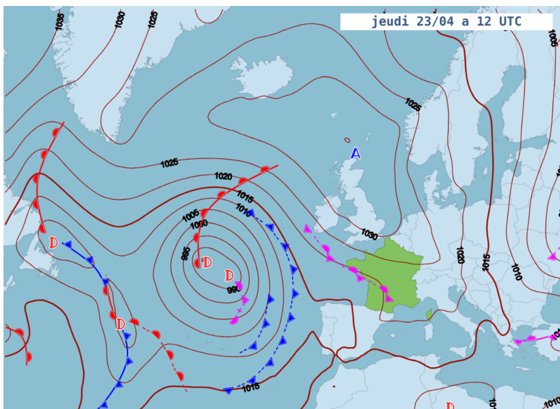
Carte des isobares au niveau de la mer et des fronts prévue pour le jeudi 23 avril à 14H00 locales
